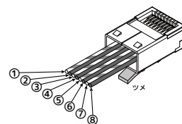
RJ45 コネクタの配線 (T568B 結線)
