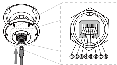
底面部の RJ45 コネクタにケーブルを差し込みます (イーサネットポートには接続しないでください)
