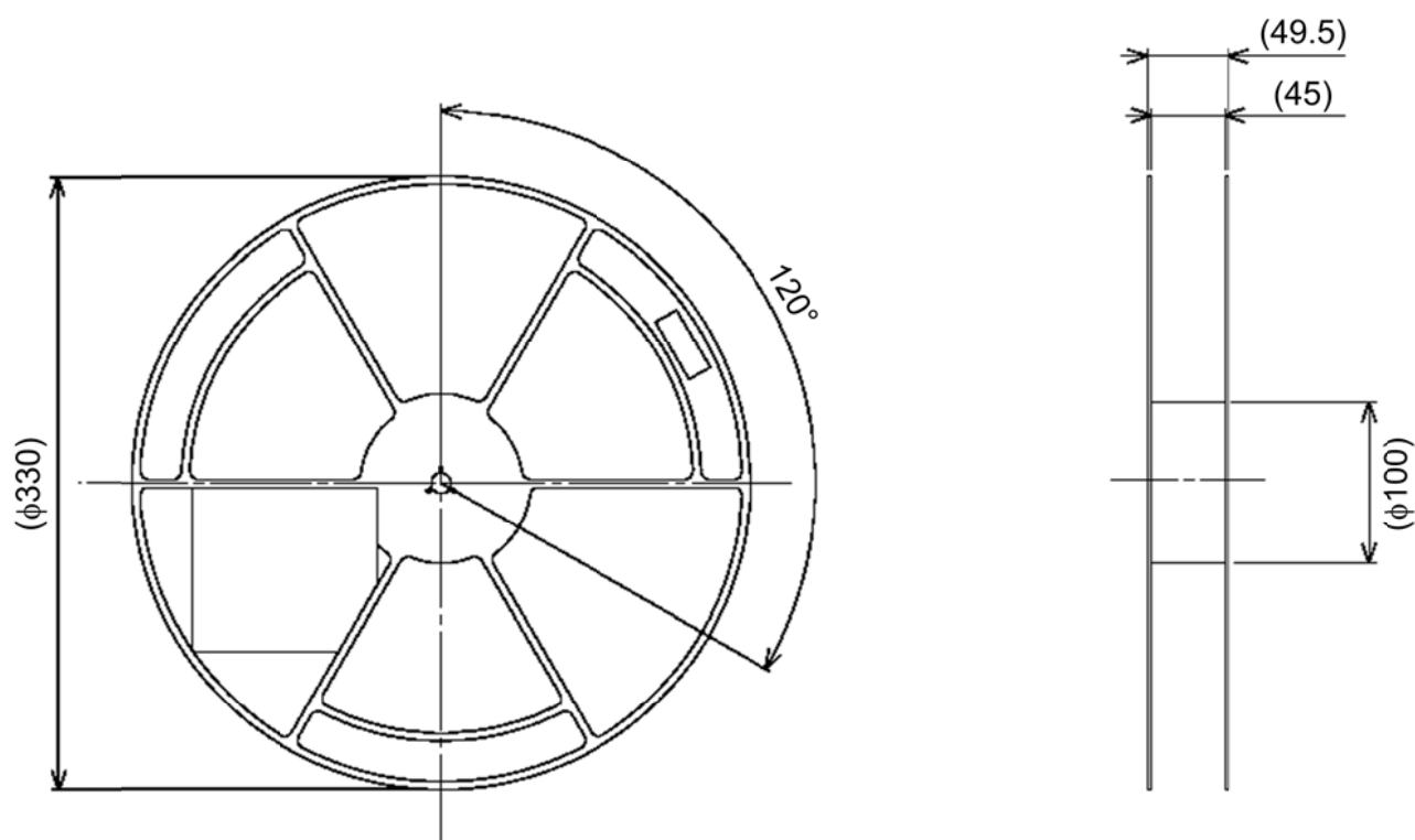
Figure 13: リール寸法
